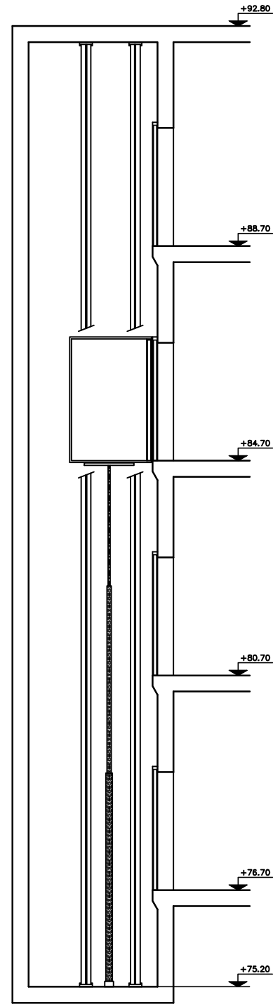
ΚΑΤΑΚΟΡΥΦΗ ΤΟΜΗ ΦΡΕΑΤΟΣ ΚΩΔΙΚΑΣ 1:50
