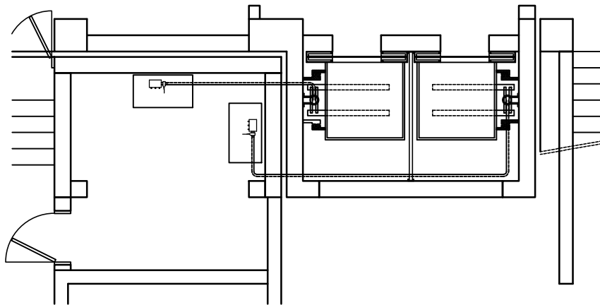
ΚΑΤΟΨΗ ΜΗΧΑΝΟΣΤΑΣΙΟΥ ΚΩΔΙΚΑΣ 1:50
