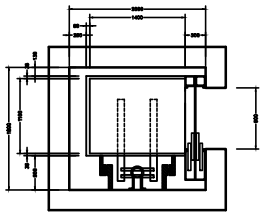
ΟΡΙΖΟΝΤΙΑ ΤΟΜΗ ΦΡΕΑΤΟΣ ΑΝ-3 , ΑΝ-4 ΚΛΙΜΑΚΑ 1:50
