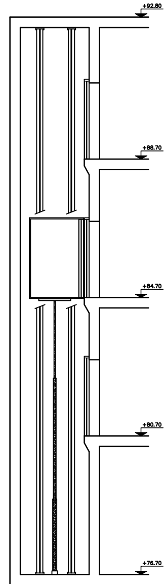
ΚΑΤΑΚΟΡΥΦΗ ΤΟΜΗ ΦΡΕΑΤΟΣ ΑΝ-3 , ΑΝ-4 ΚΛΙΜΑΚΑ 1:50
