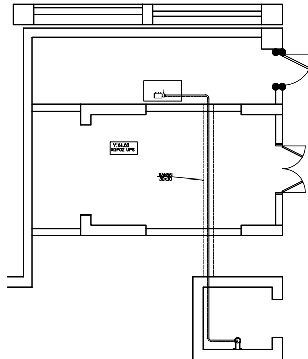
ΚΑΤΟΨΗ ΜΗΧΑΝΟΣΤΑΣΙΟΥ ΑΝ-4 ΚΛΙΜΑΚΑ 1:50
