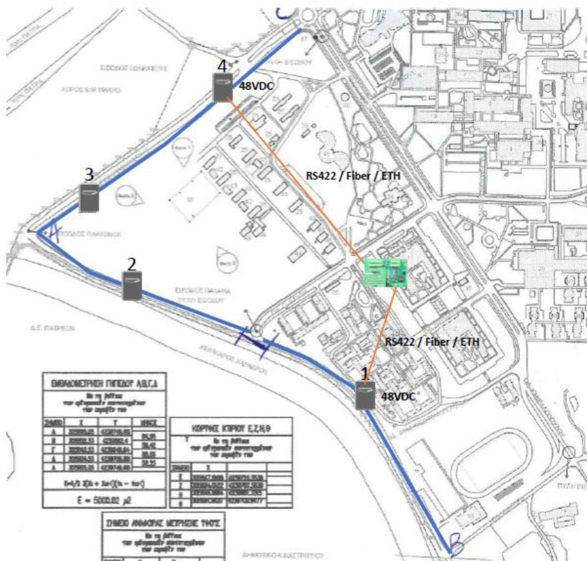
Εικόνα 1. Ενδεικτική περιοχή κάλυψης του συστήματος προστασίας.
