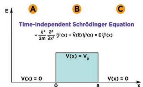
Εικόνα 2: Η εξίσωση Schrödinger και ένα φράγμα με ύψος V_0 . Η συνάρτηση \psi είναι η λύση της εξίσωσης Schrodinger. (Η εικόνα πάρθηκε από το κανάλι στο YouTube, Professor Dave explains).
