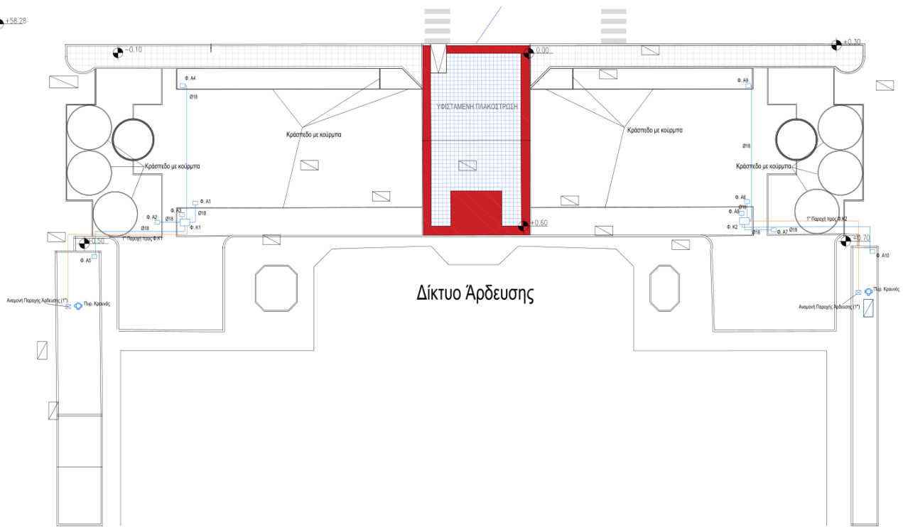
Εικόνα 4 - Δίκτυο Άρδευσης
