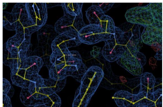
Ηλεκτρονιακή πυκνότητα
