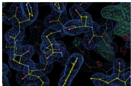
Ηλεκτρονιακή πυκνότητα
