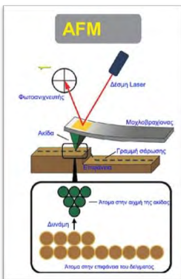
Τυπική διάταξη λειτουργίας του AFM
