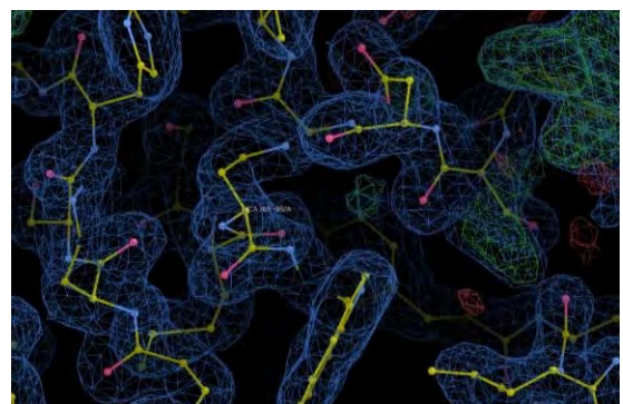
Ηλεκτρονική πυκνότητα
